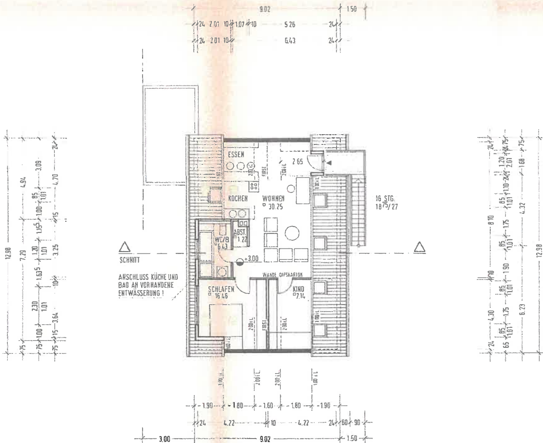
DACHGESCHOSS
