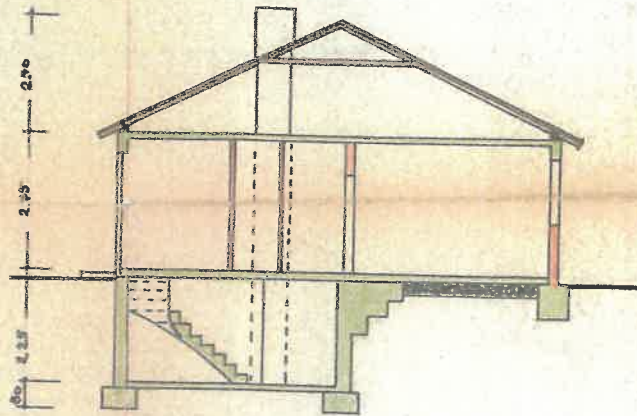
SCHNITT
